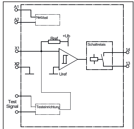
Prinzipialschaltbild ELMON relay 31-30
