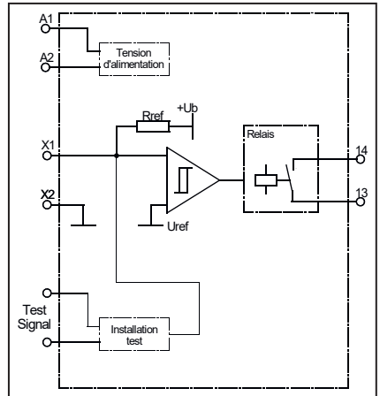
Schéma de principe du ELMON relay 31-30
